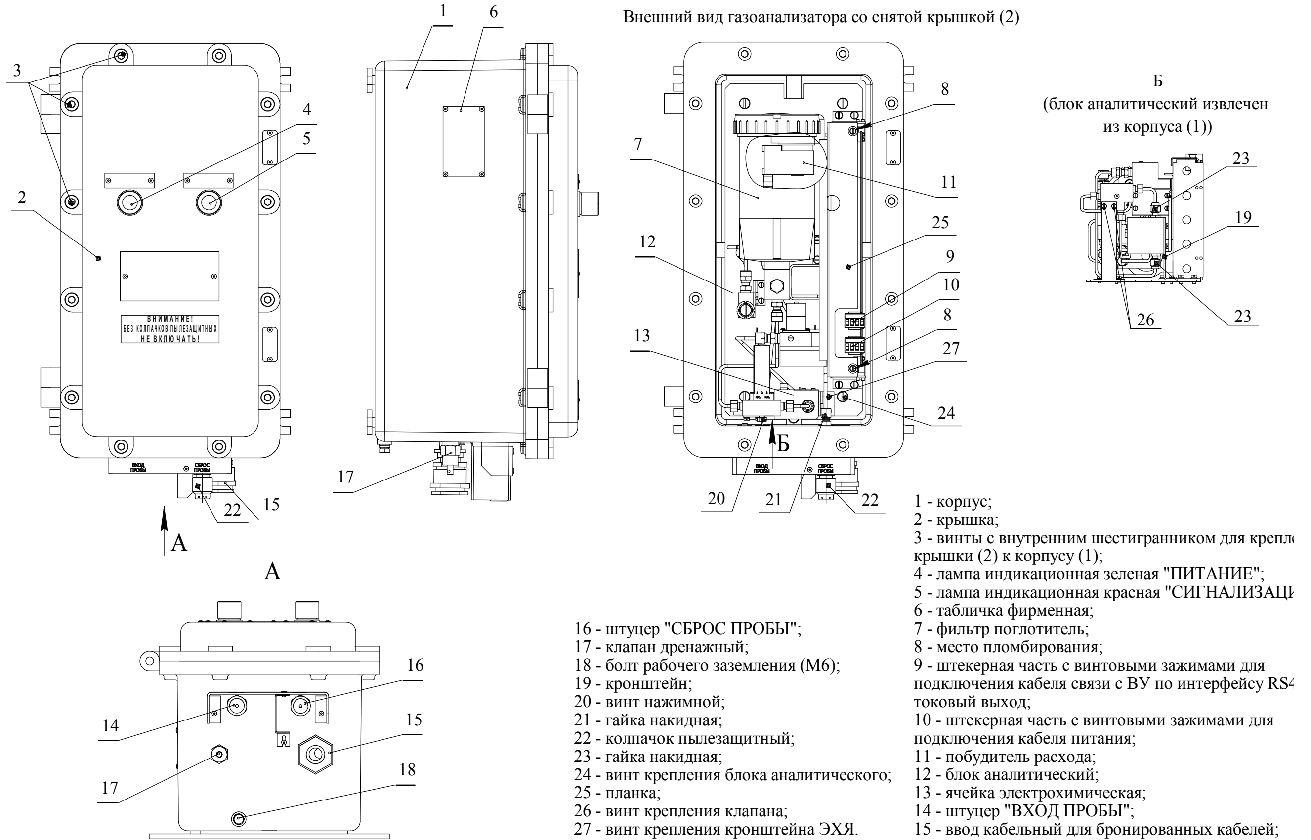
Рисунок 1.1 – Датчик-газоанализатор паров КРТ ДАРТ. Внешний вид
